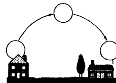
Полнолуние
